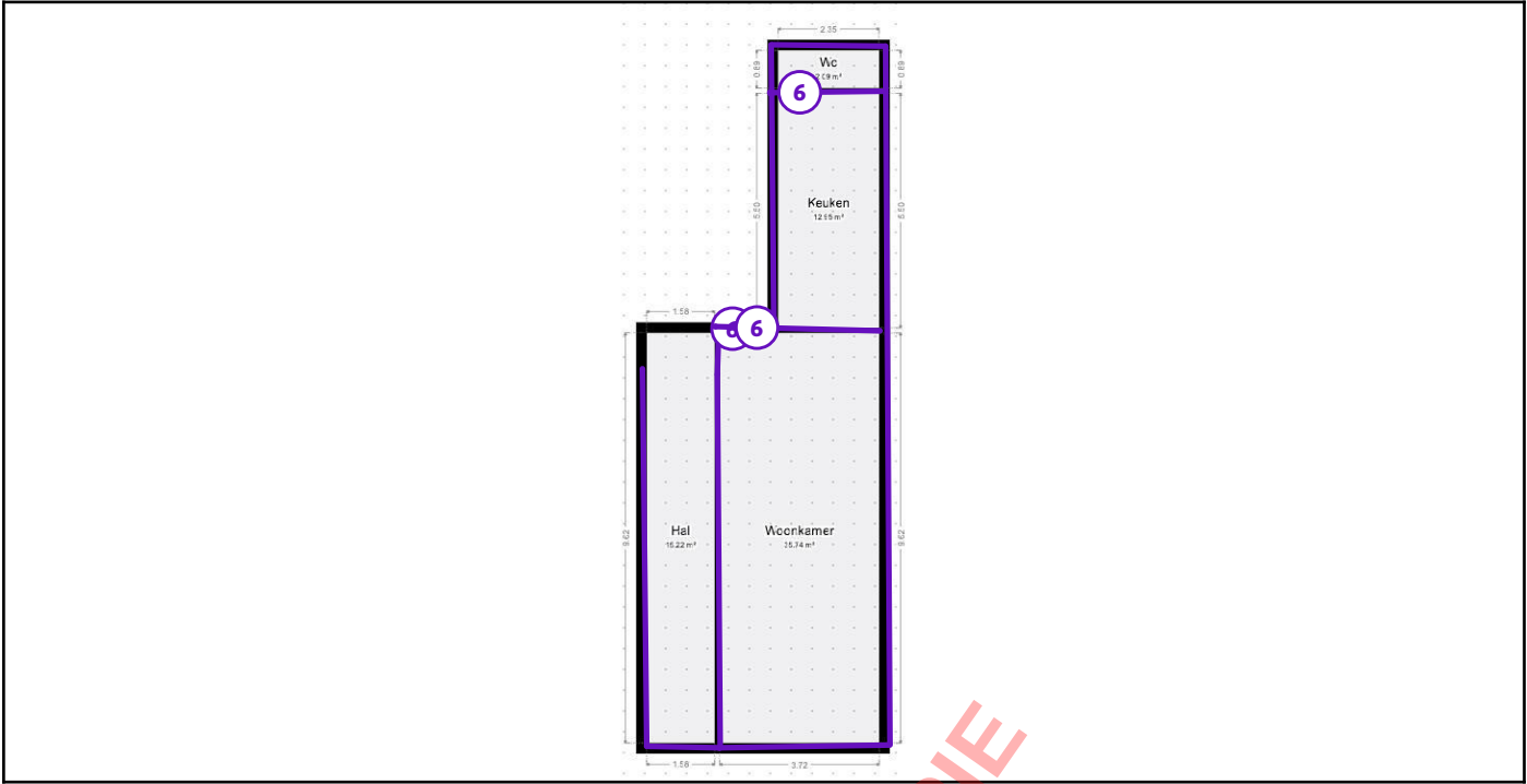
Legende van plan 1.3: Grondplan +0
