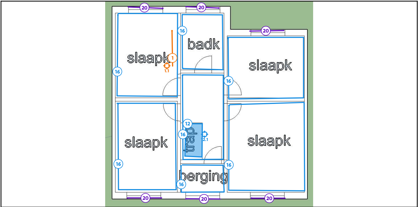
Legende van plan 1.5: plan 1ste verdieping wanden en varia
