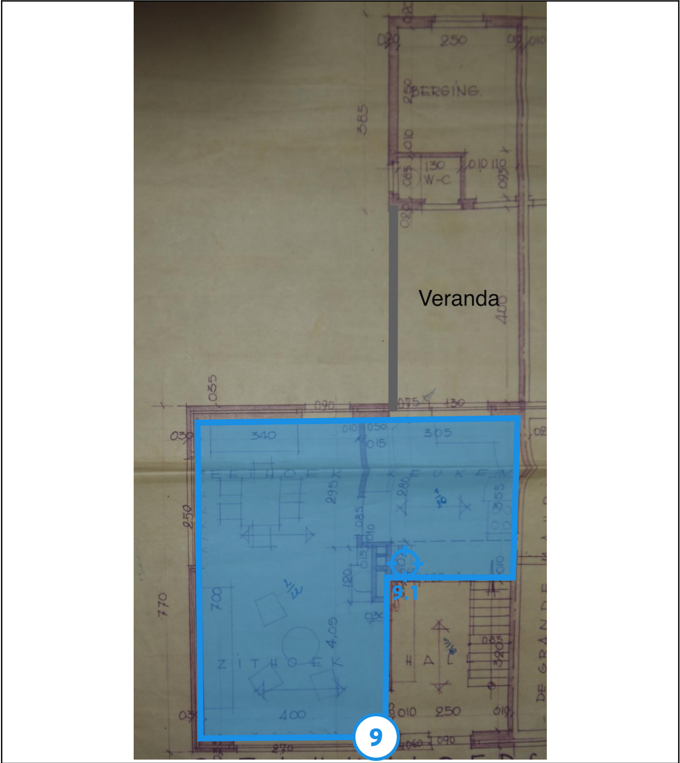
Legende van plan 1.4: Grondplan - Gelijkvloers
